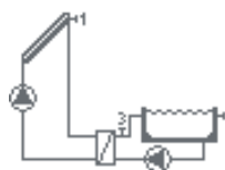
Solární systém s tepelným výměníkem a bazénem
